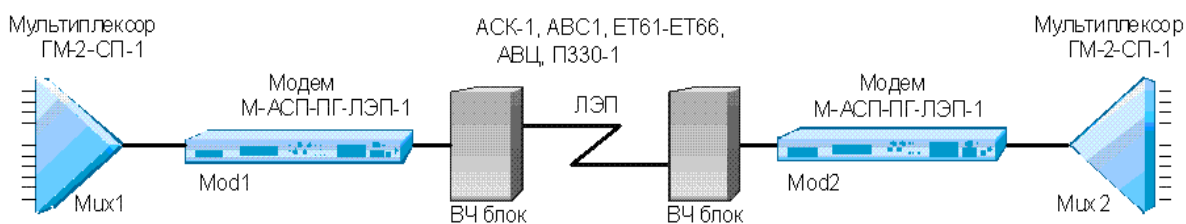
Рис.28. Организация связи между мультиплексорами через модемы М-АСП-ПГ-ЛЭП
