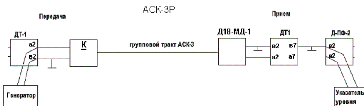
Рис.1. Схема измерения АЧХ в АСК-3Р.
