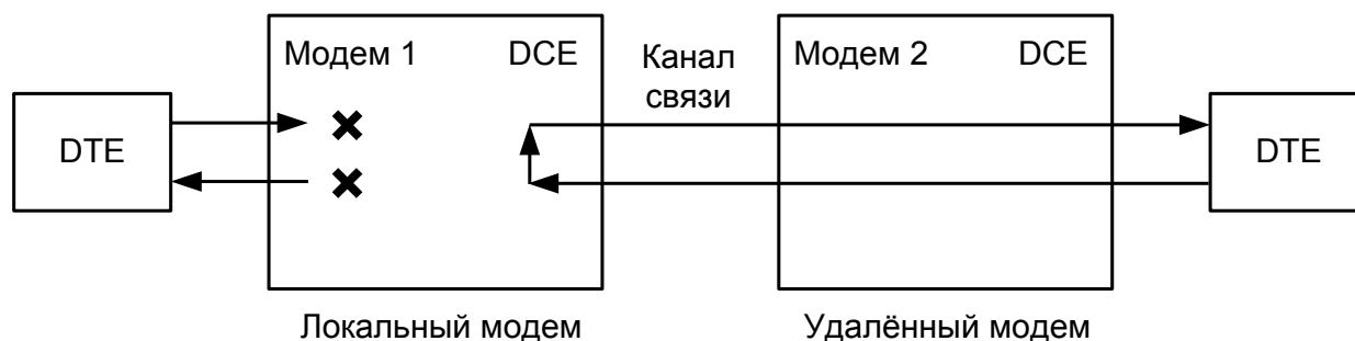
Рис.18. Проверка в режиме DL — “цифровой шлейф”
