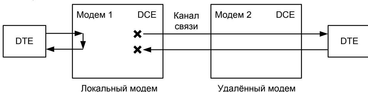
Рис.32. Проверка в режиме LL — “местный цифровой шлейф”
