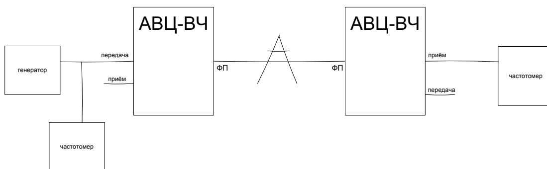
Рис.3. Схема для измерения сдвига частоты в групповом тракте.
