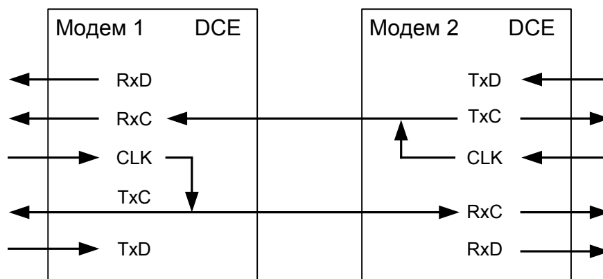
Рис.24. Синхронизация в режиме External модема 2 (модем 1 — синхронизация External).
