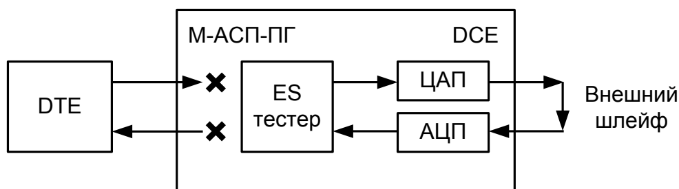
Рис.15. Проверка в режиме подключения ES-тестера к каналу связи
