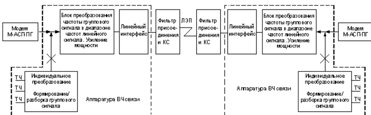
Рис. 8. Схема подключения модемов для организации дуплексного канала связи
