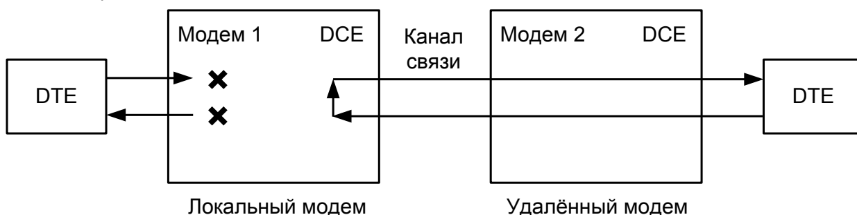
Рис.31. Проверка в режиме DL — “цифровой шлейф”
