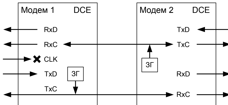
Рис. 20. Синхронизация в режиме Internal модема 2 (модем 1 — синхронизация Internal)
