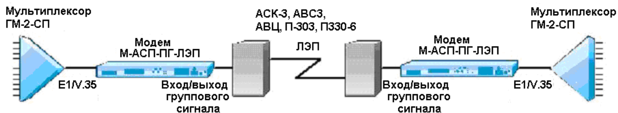
Рис. 1. Подключение модемов М-АСП-ПГ-ЛЭП к аппаратуре ВЧ связи по ЛЭП в цифровом и аналоговом режиме работы комплекса К-ЛЭП.
