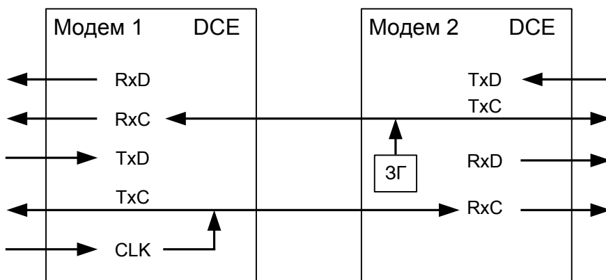
Рис.23. Синхронизация в режиме Internal модема 2 (модем 1 — синхронизация External).
