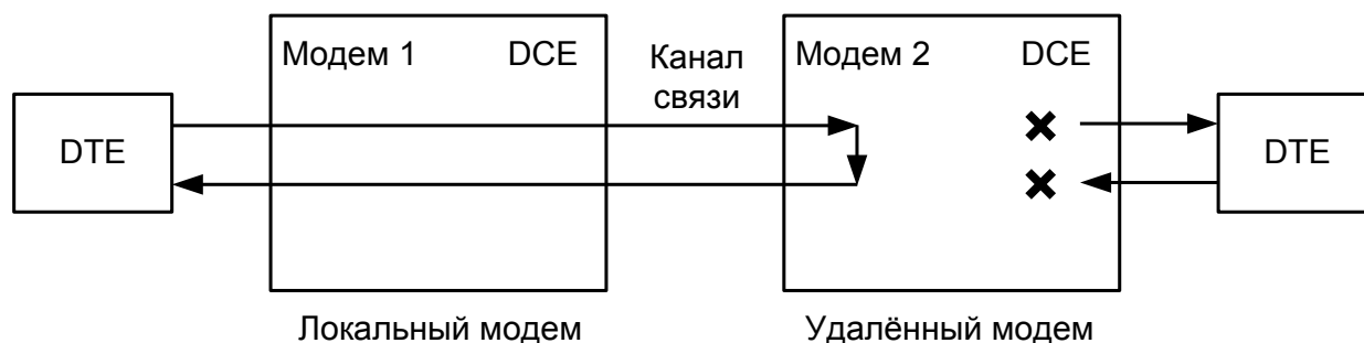
Рис.16. Проверка в режиме RDL “удаленный цифровой шлейф”.
