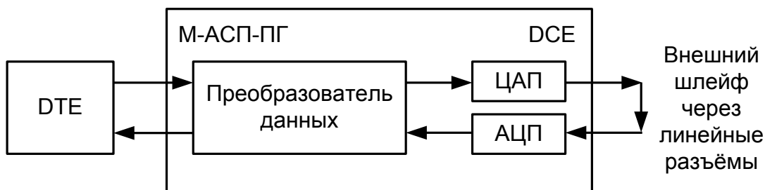
Рис.17. Проверка в режиме AL — “Аналоговый шлейф”
