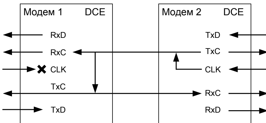
Рис.27. Синхронизация в режиме External модема 2 (модем 1 — синхронизация Receiver).
