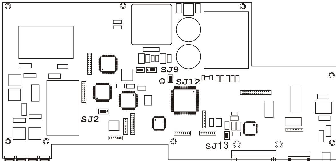
Рис. 7. Расположение элементов на плате модема М-АСП-ПГ-ЛЭП
