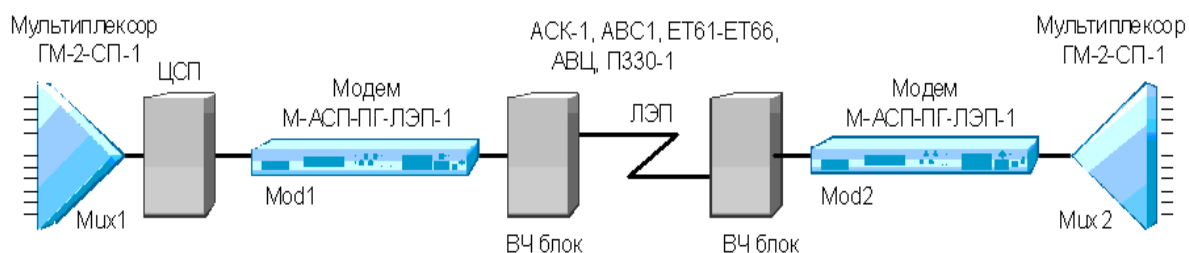
Рис.29. Организация связи между мультиплексором и модемом через ЦСП
