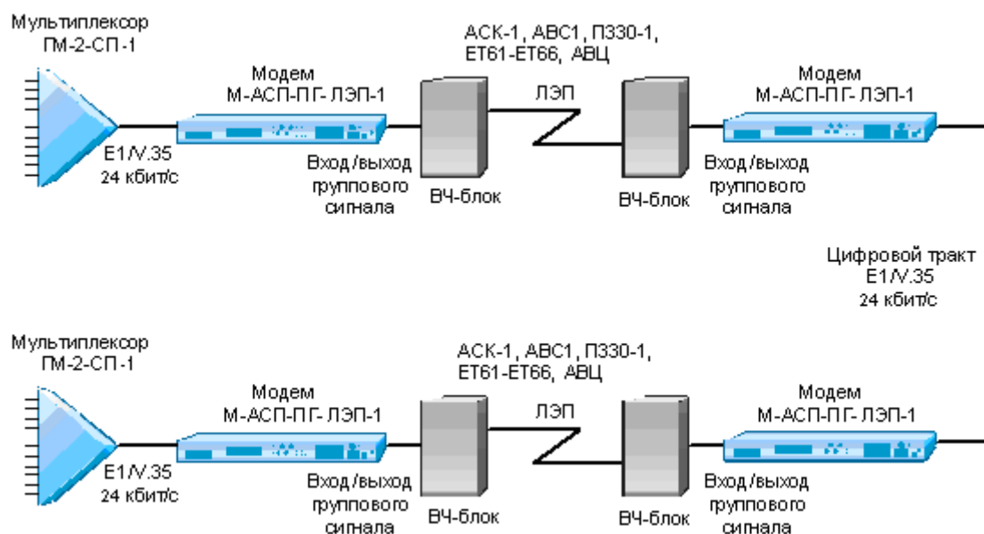
Рис. 1. Подключение модемов М-АСП-ПГ-ЛЭП к аппаратуре ВЧ связи по ЛЭП в цифровом и аналоговом режиме работы комплекса К-ЛЭП.
