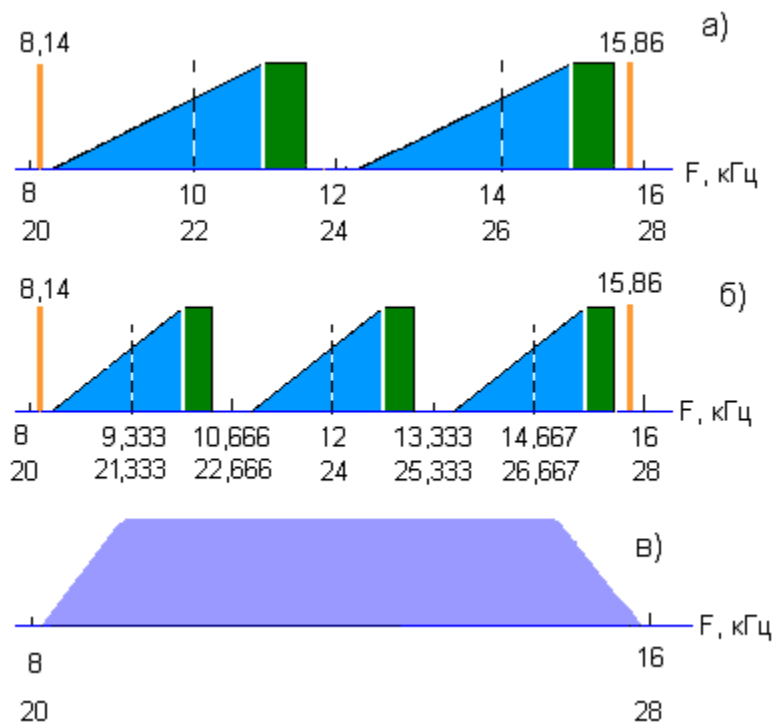
Рис.5. Расположение спектра группового сигнала для системы передачи с шириной полосы частот 8 кГц (аналоговый и цифровой режим).
