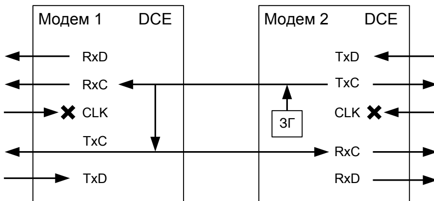
Рис.26. Синхронизация в режиме Internal модема 2 (модем 1 — синхронизация Receiver).
