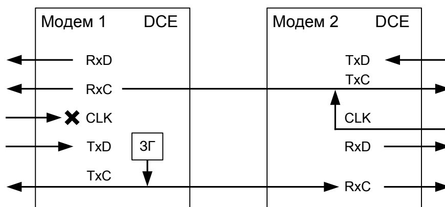
Рис.21. Синхронизация в режиме External модема 2 (модем 1 — синхронизация Internal)
