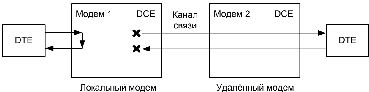
Рис.19. Проверка в режиме LL — “местный цифровой шлейф”
