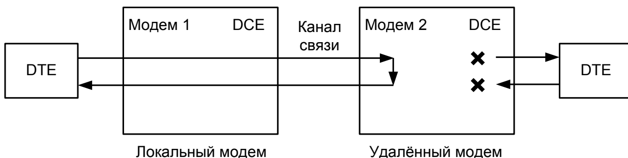
Рис. 30. Проверка в режиме RDL “удаленный цифровой шлейф”.
