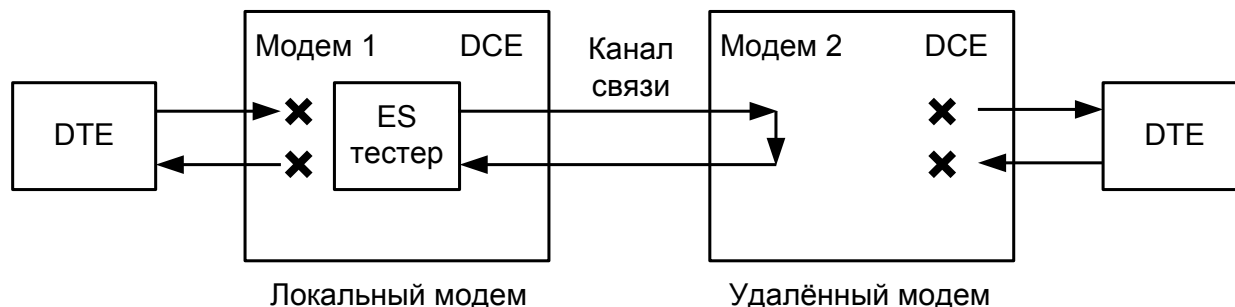
Рис. 13. Проверка в режиме RDL-ES — «удаленный шлейф» с использованием ES-тестера
