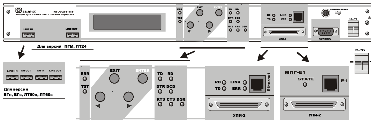
Рис. 6. Передняя панель модема М-АСП-ПГ-ЛЭП, М-АСП-ПГ-ЛЭП-1 и М-АСП-ПГ-ЛЭП-2.
