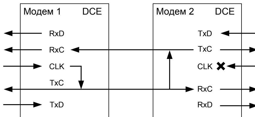
Рис.25. Синхронизация в режиме Receiver модема 2 (модем 1 — синхронизация External).
