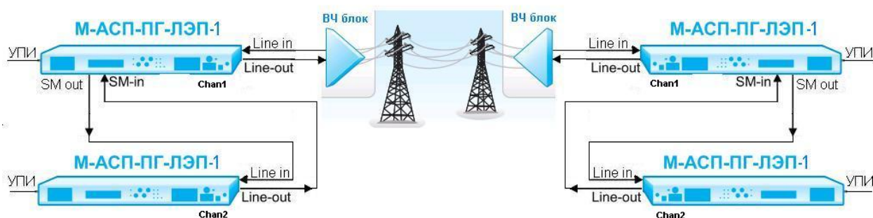
Рис. 9. Схема подключения двух модемов М-АСП-ПГ-ЛЭП-1 при работе через ВЧ блок с шириной полосы частот тракта 8 кГц.
