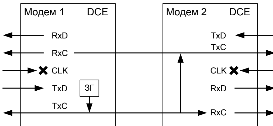
Рис.22. Синхронизация в режиме Receiver модема 2 (модем 1 — синхронизация Internal).
