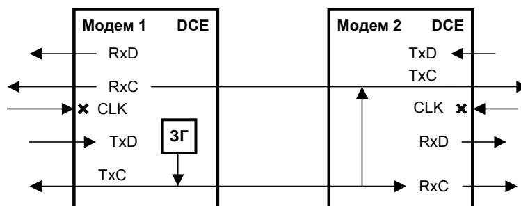
Рис. 40. Синхронизация в режиме Receiver модема 2
