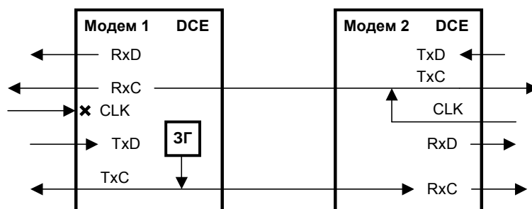
Рис. 39. Синхронизация в режиме External модема 2
