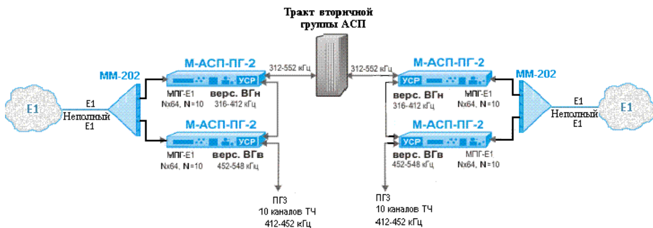
Рис. 27. Передача 20-ти КИ потока Е1 через тракт ВГ со скоростью 1280 кбит/с с помощью двух пар модемов М-АСП-ПГ-2.
