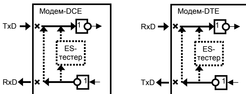
Рис. 46. Включение инверторов для цепей RxD и TxD в тестовых режимах RDL/AL-ES, DL.
