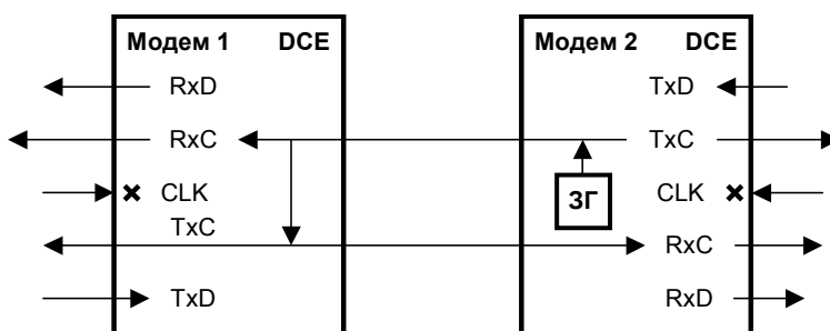
Рис. 44. Синхронизация в режиме Internal модема 2.
