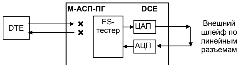
Рис. 32. Проверка в режиме AL-ES - «Аналоговый шлейф» с использованием ES-тестера
