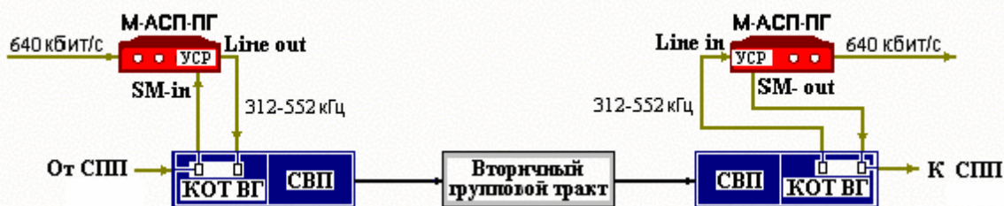
Рис. 18. Схема подключения модемов версии ВГн (ВГв) к ВГТ при совместной передаче сигналов данных со скоростью до 640 кбит/с и сигналов каналов ТЧ.
