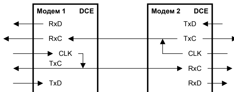
Рис. 42. Синхронизация в режиме External модема 2.
