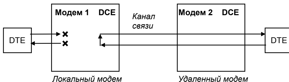
Рис. 36. Проверка в режиме DL - «цифровой шлейф»
