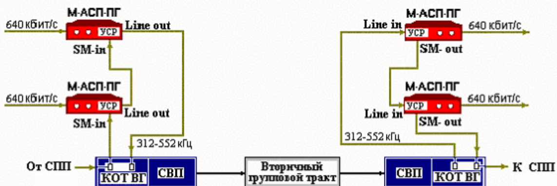
Рис. 17. Схема подключения двух пар модемов версий ВГн и ВГв к ВГТ при совместной передаче сигналов данных со скоростью до 1280 кбит/с и сигналов каналов ТЧ.
