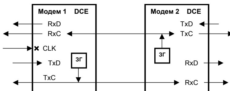
Рис. 38. Синхронизация в режиме Internal модема 2
