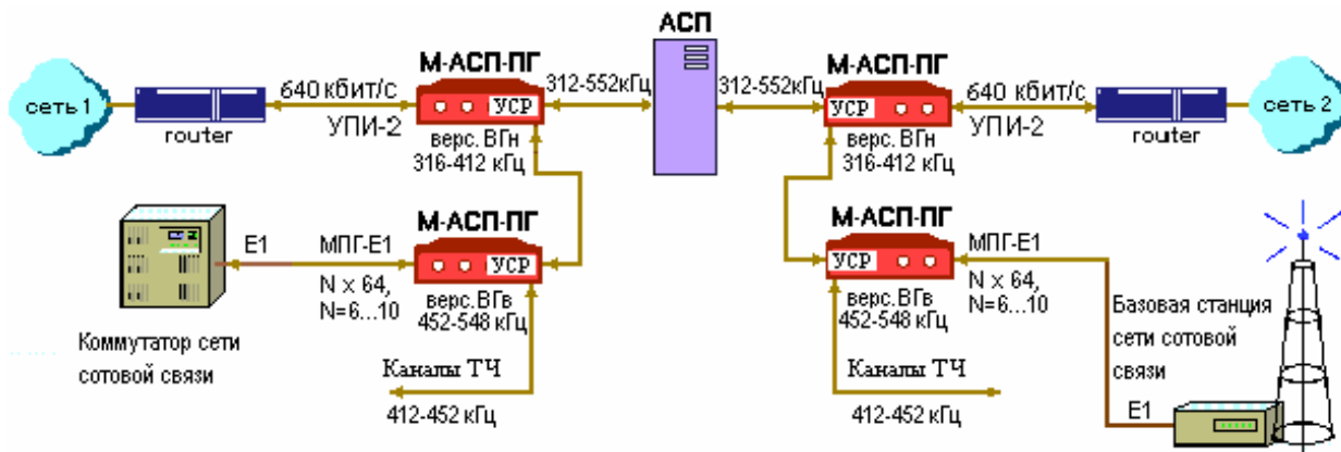
Рис. 11. Включение одной пары модемов (версии ВГн или ВГв) в тракт вторичной группы и подключение к АТС с помощью интерфейсного модуля МПГ-Е1.
