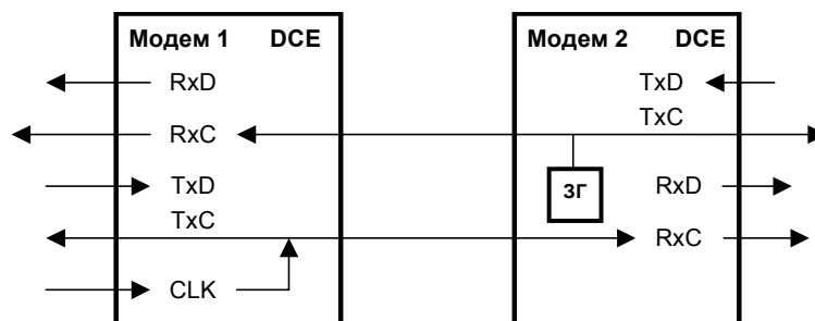
Рис. 41. Синхронизация в режиме Internal модема 2.
