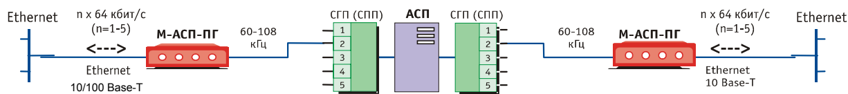
Рис. 3. Пример объединения сетей Ethernet 10/100 Base-T с помощью модема М-АСП-ПГ (версия ПГМ).
