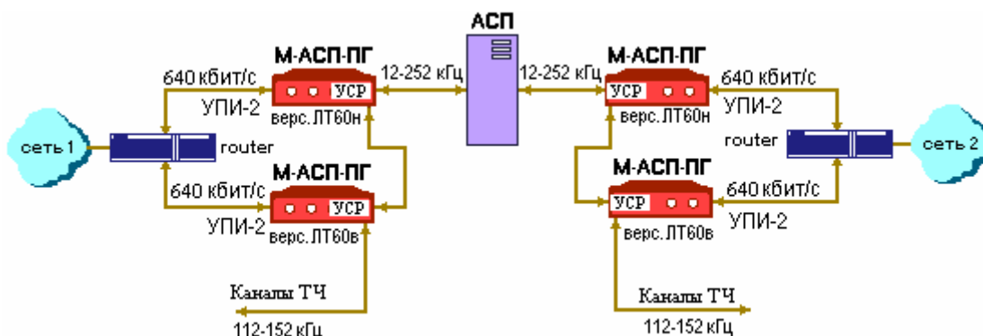
Рис. 7. Использование двух пар модемов (версии ЛТ60н и ЛТ60в) для передачи цифрового потока со скоростью 1280 кбит/с по линейному тракту АСП К-60П.
