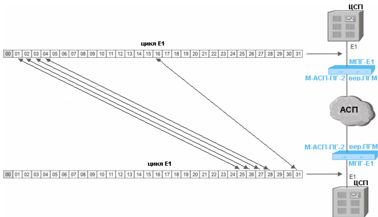
Рис. 27. Передача 20-ти КИ потока Е1 через тракт ВГ со скоростью 1280 кбит/с с помощью двух пар модемов М-АСП-ПГ-2.
