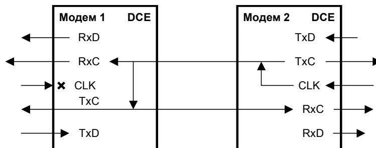
Рис. 45. Синхронизация в режиме External модема 2.
