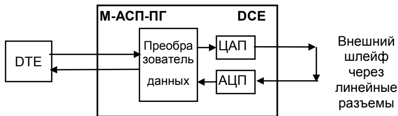
Рис. 35. Проверка в режиме AL- «Аналоговый шлейф»
