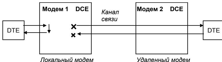
Рис. 37. Проверка в режиме LL - «местный цифровой шлейф»
