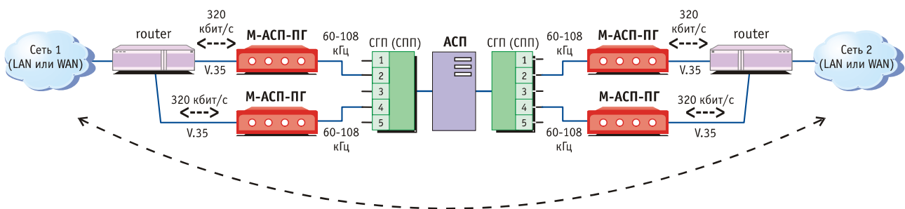
Рис. 3. Пример объединения сетей Ethernet 10/100 Base-T с помощью модема М-АСП-ПГ (версия ПГМ).
