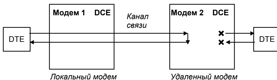
Рис. 34. Проверка в режиме RDL “удаленный цифровой шлейф”.
