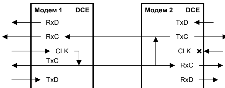
Рис. 43. Синхронизация в режиме Receiver модема 2.
