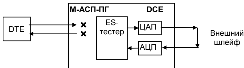
Рис. 33. Проверка в режиме подключения ES-тестера к каналу связи
