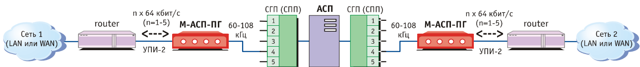
Рис. 2. Пример подключения ООД по интерфейсу УПИ-2 к модему М-АСП-ПГ (версия ПГМ).
