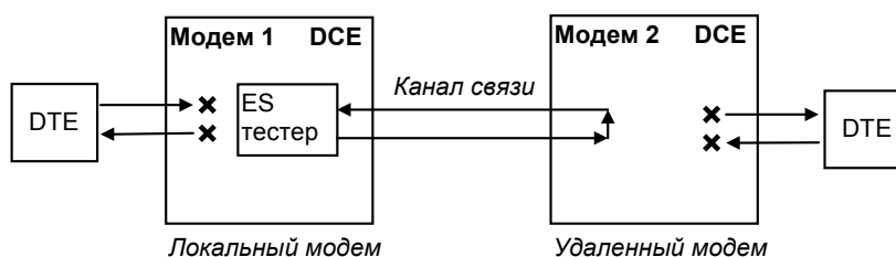
Рис. 31. Проверка в режиме RDL-ES - «удаленный шлейф» с использованием ES-тестера
