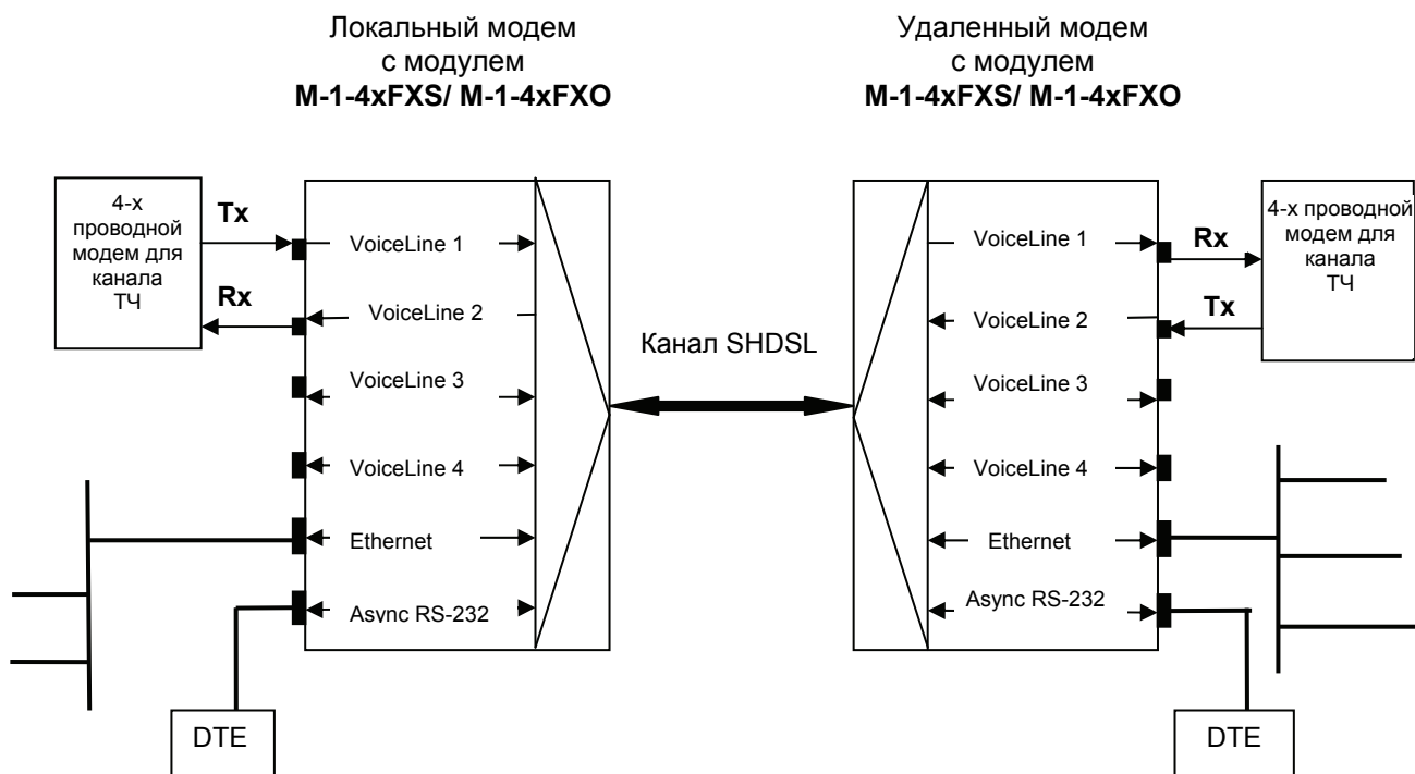
Рис. 16 Схема включения 4-проводного модема для каналов ТЧ в сеть передачи данных образованную двумя модемами Зелакс DSL М-1Д
