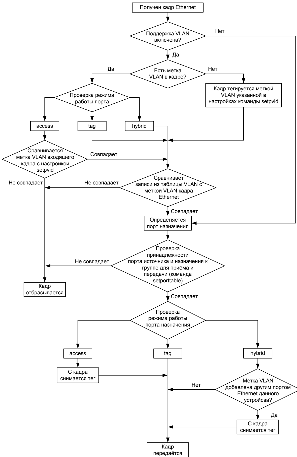
Рис. 11. Алгоритм работы портов Ethernet
